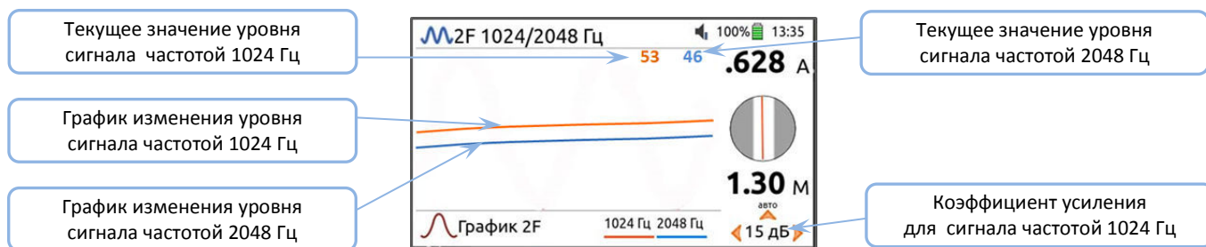
Рисунок 3.15. Режим индикации «График 2F».
