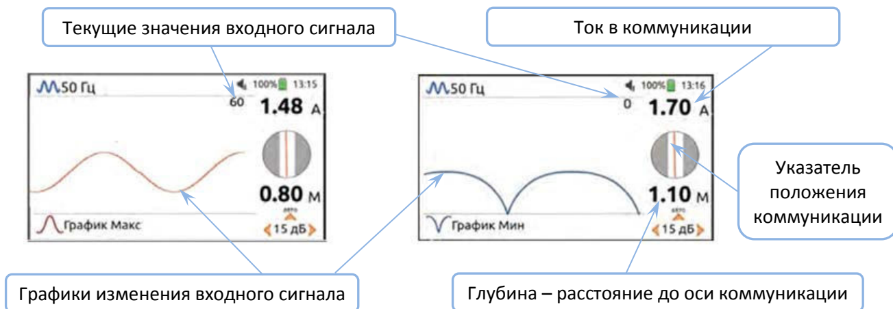
Рисунок 3.12. Режимы «График Макс» и «График Мин».
