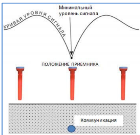
Рисунок 3.9. Метод «минимума».
