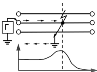
Рисунок Б.1. КЗ-однофазное.
