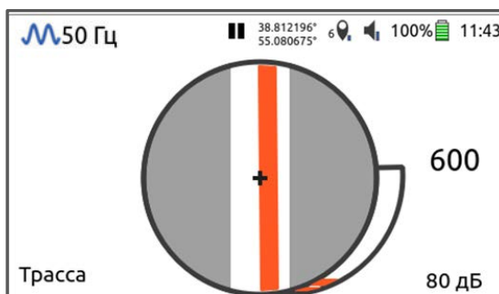
Рисунок 5.6. Вид экрана в режиме «Пауза» .
