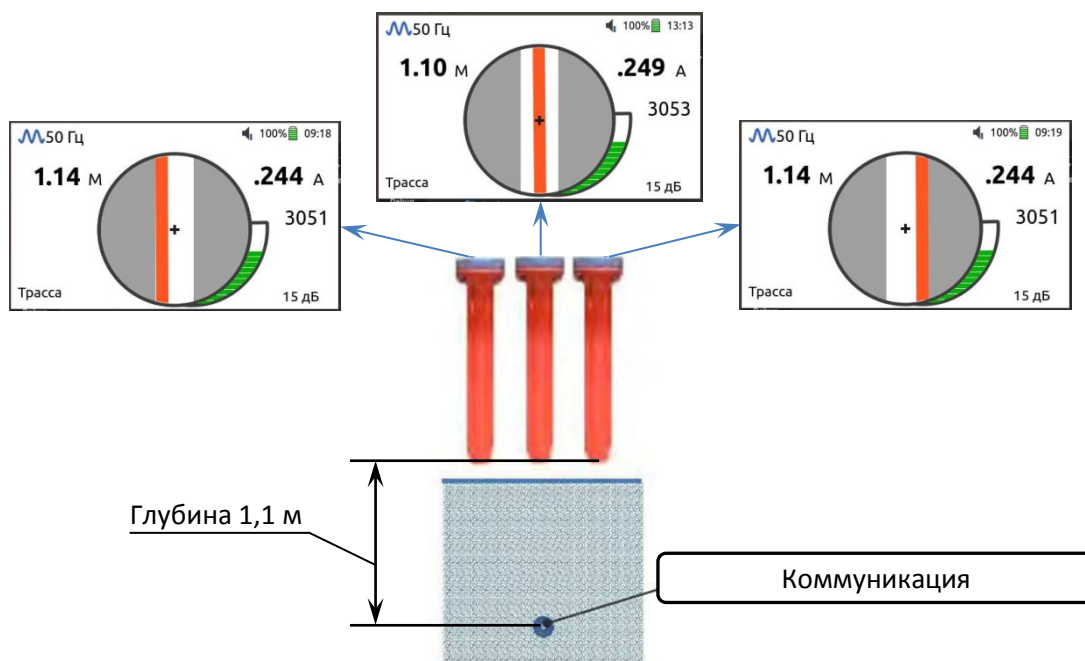
Рисунок 3.6. Измерение глубины залегания коммуникации.
