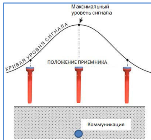
Рисунок 3.10. Метод «максимума».
